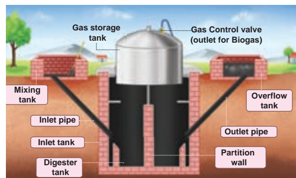
Fig. 8.3 Biogas Unit
